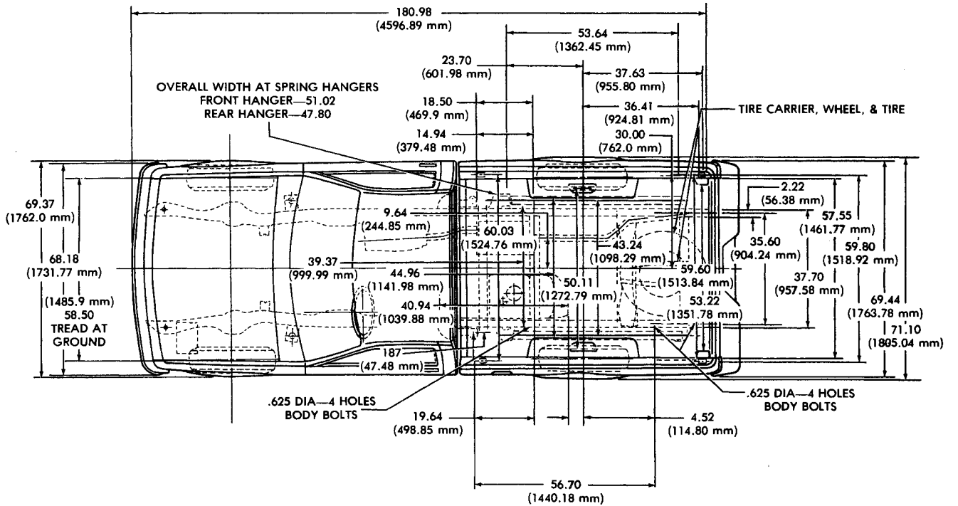
Fig. 2—Dakota Dimensions
